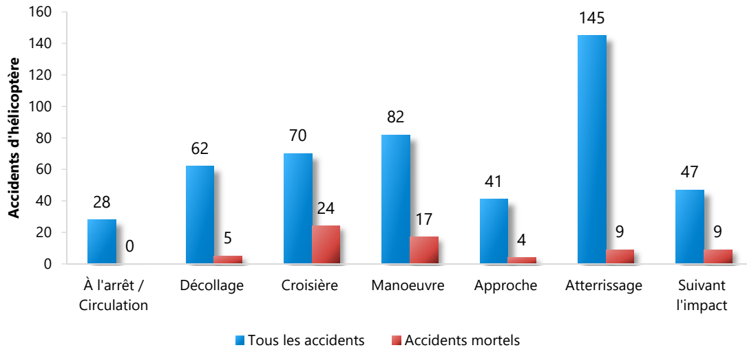
Figure 7. Accidents d'hélicoptère et accidents mortels comportant des événements durant des phases de vol précises, 2009 à 2019
