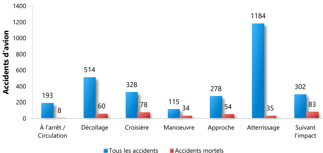
Figure 6. Accidents d'avion et accidents mortels comportant des événements durant des phases de vol précises, 2009 à 2019
